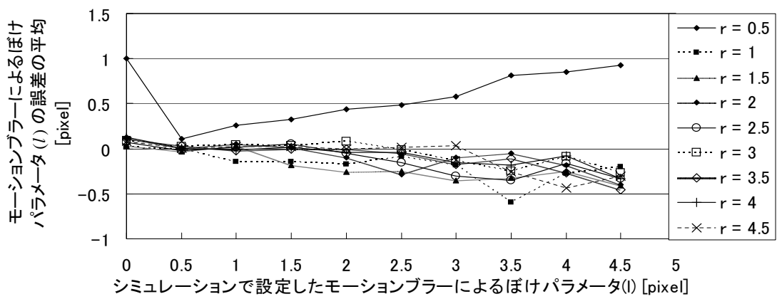
(b) 様々な r, \theta の元での推定された PSF パラメータ l の真値に対する誤差 .
