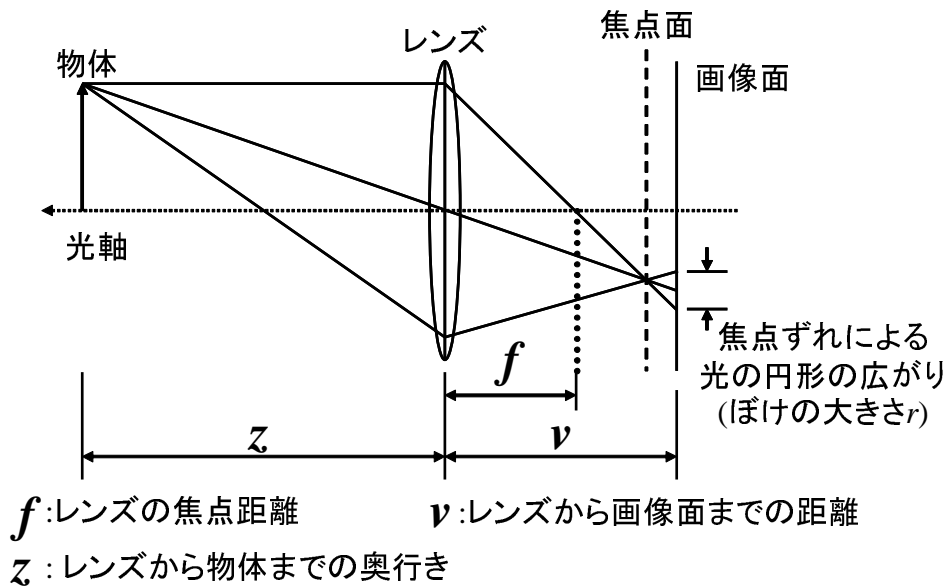
図 11 焦点ずれが生じている場合の光学系
