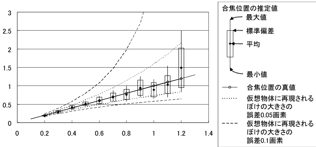
図 30 手で設定した合焦位置と推定された合焦位置の関係
