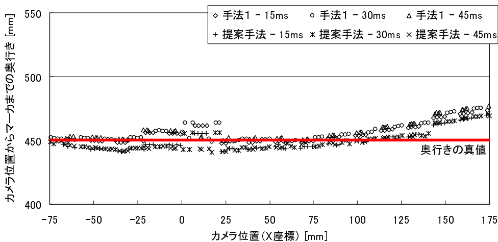
図 22 複数のマーカを用いて推定されたカメラからマーカまでの奥行き
