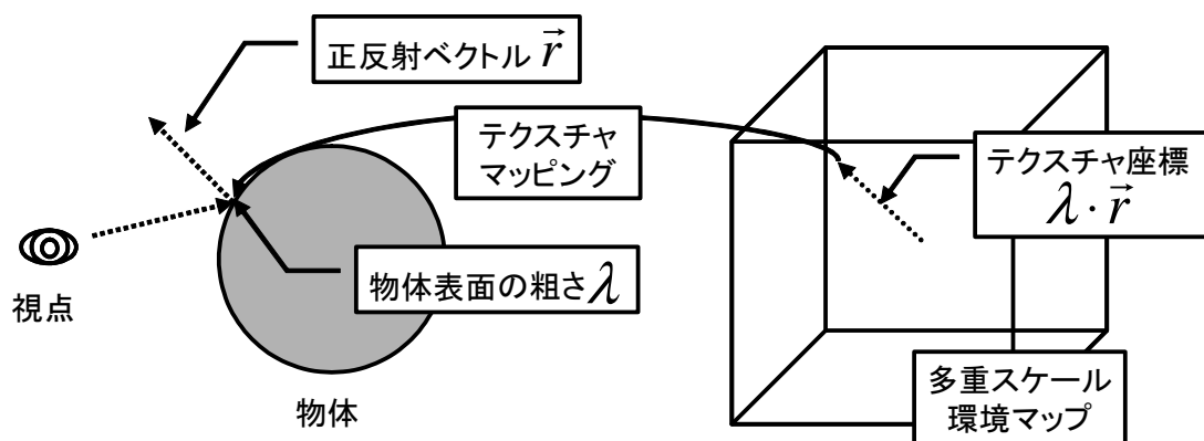
図 28 テクスチャマッピングによる写り込みの描画
