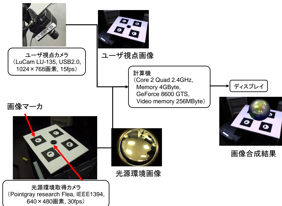
図 36 試作した拡張現実感システムの外観
