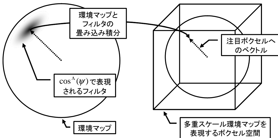
図 26 多重スケール環境マップの計算
