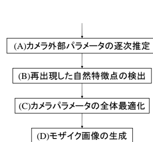
図 1: 処理の流れ
